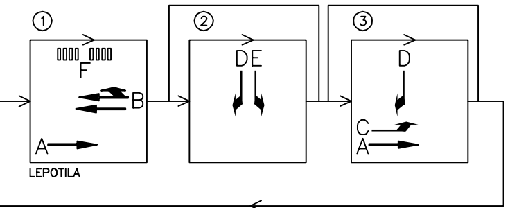
LIKENNEVALOJEN VIHREIDEN TILOJEN VAIHEKAAVIO
