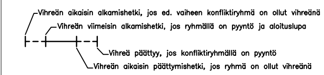
VAIHEKAAVIO
